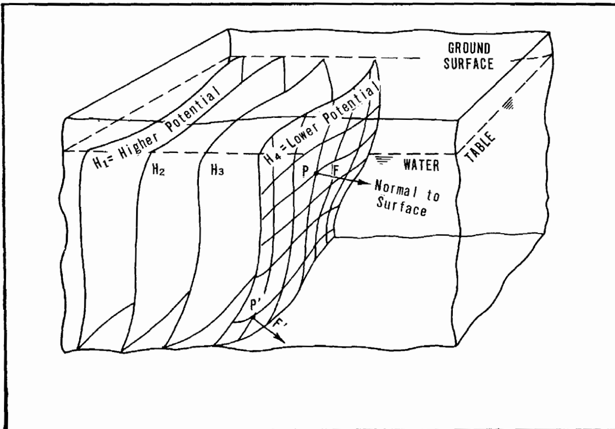
Figure 1-3, Equipotential surfaces
